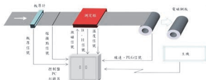
鐵損計(線上磁性量測)
