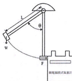
圖 1 衝擊測試
