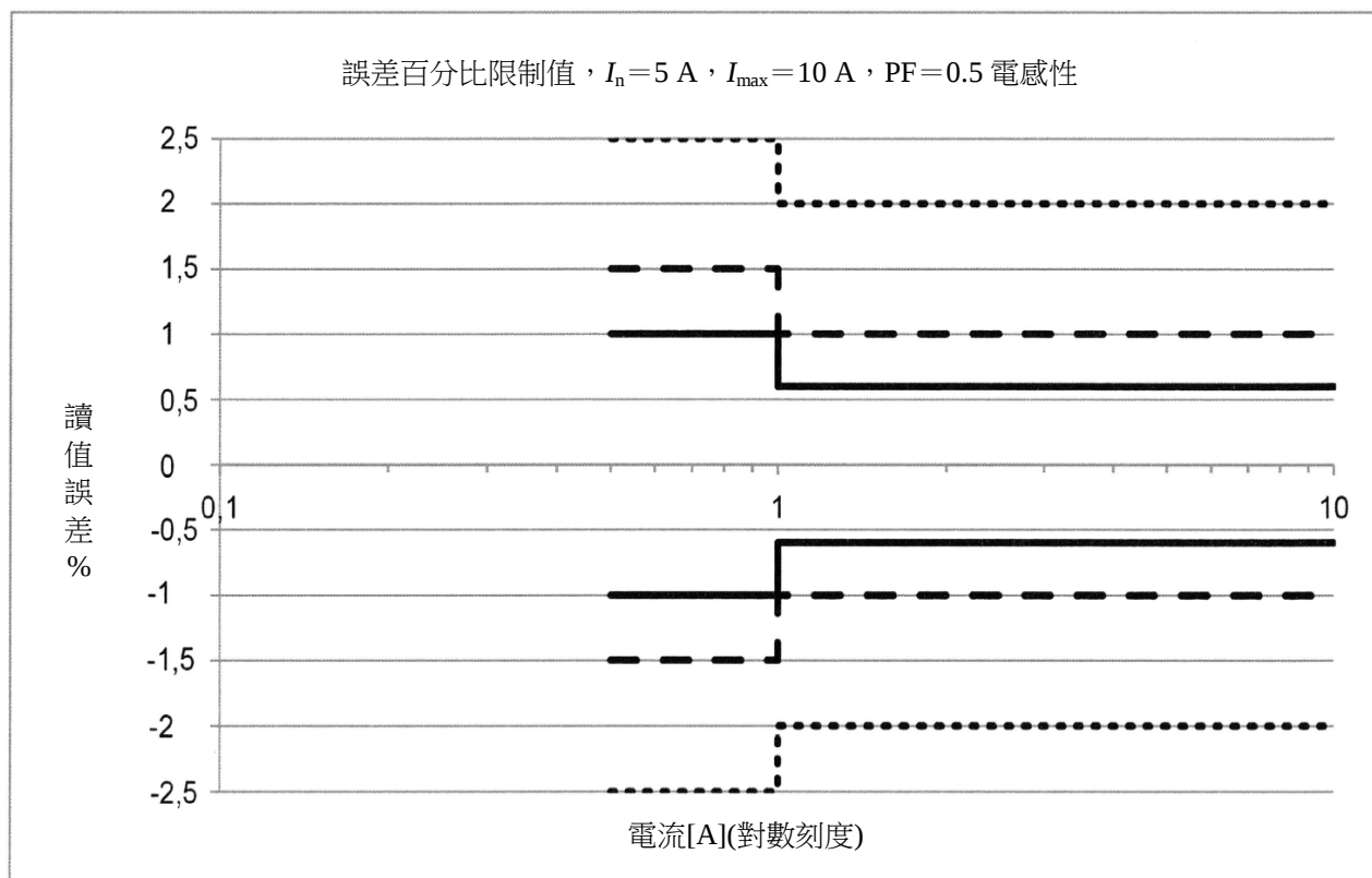
圖 A. 2 0.5 級、1 級及 2 級瓦時計之允收誤差百分比限制值的比較
