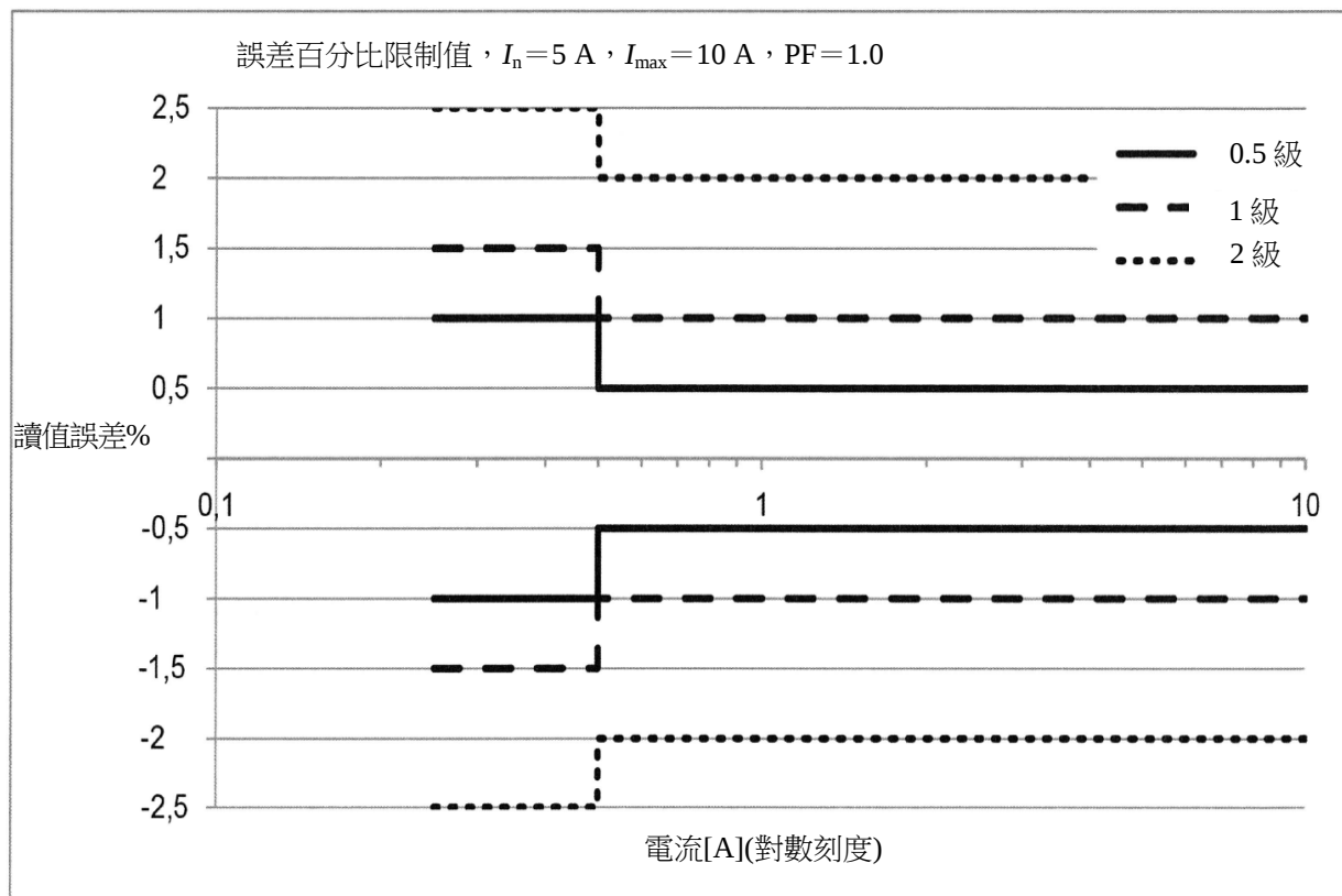
圖 A.1 0.5 級、1 級及 2 級瓦時計之允收誤差百分比限制值的比較 ( I_n = 5\text{ A} ， I_{\max} = 10\text{ A} ， \text{PF} = 1.0 ，用於直接連接)
