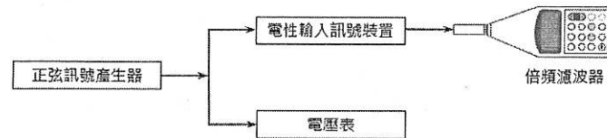
圖 1 倍頻濾波器平坦頻率響應檢測系統圖
