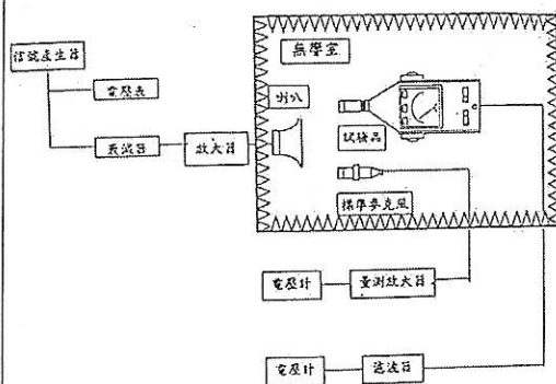
噪音計的器差測試系統圖
