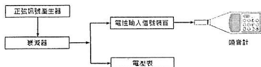
圖 7 噪音計位準線性度檢測系統
