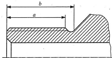
圖 B.2 螺紋
