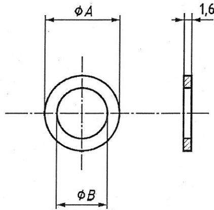
圖 A.7 螺紋型干擾產生器之襯墊
