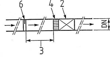
測試 5A 附加整流器之配置
