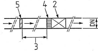
測試 3A 附加整流器之配置
