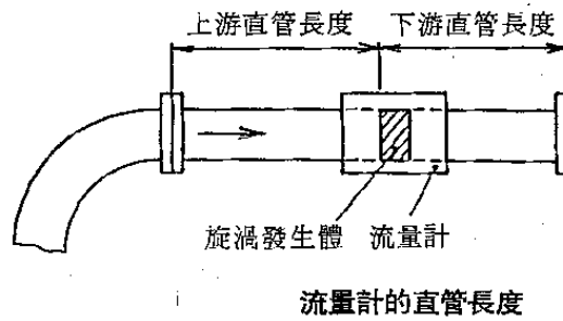
流量計上游處之各類接頭與流量計間之必要的最小直管長度
