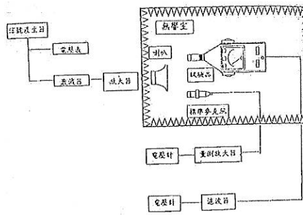
噪音計的器差測試系統圖
